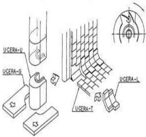
Елементи футерування
